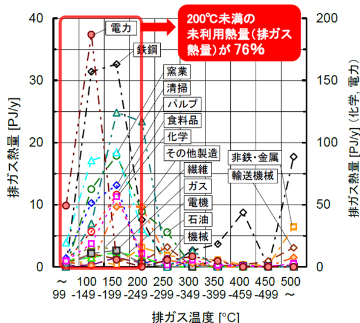
図 II -11 業種別・温度帯別の未利用熱量（排ガス熱量）の全国推定値（化学、電力は右軸） （出典：NEDO，産業分野の排熱実態調査報告書，2019， https://www.nedo.go.jp/news/press/AA5_101074.html ）
