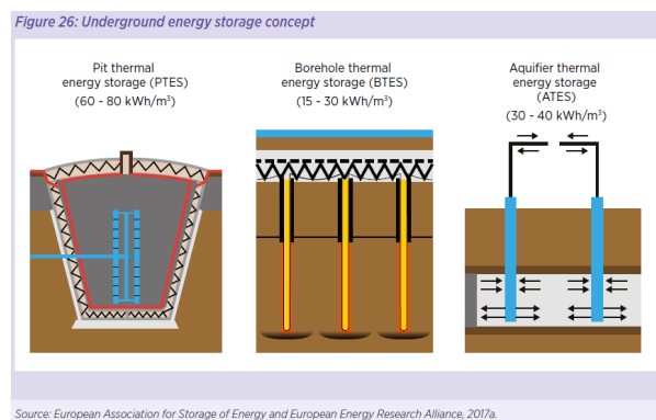
図 II -15 地下空間を利用した蓄熱システム
