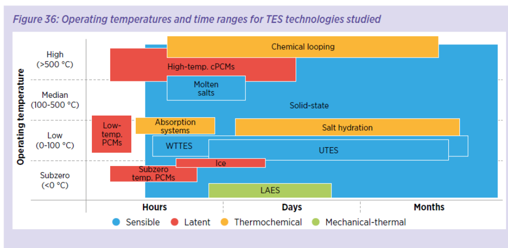
図 II -13 エネルギー部門における熱エネルギー貯蔵の利用 (出典：IRENA, Innovation Outlook Thermal Energy Storage, 2020)
