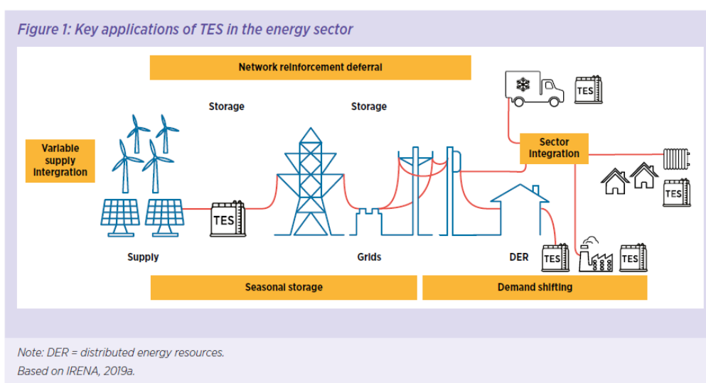
図 II -12 エネルギー部門における熱エネルギー貯蔵の利用 (出典：IRENA, Innovation Outlook Thermal Energy Storage, 2020)
