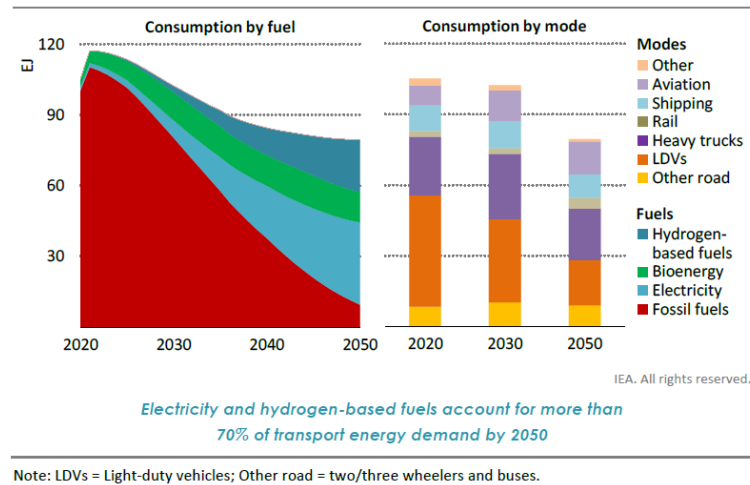
図 II-9 NET ZERO by 2050 (NZE) シナリオにおける輸送部門のエネルギー消費量の内訳 (出典：IEA, NET ZERO by 2050, 2021)
