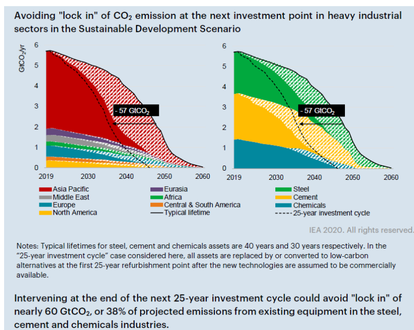
図 II-7 鉄鋼、セメント、化学工業の CO 2 排出量削減シナリオ (出典：IEA, Energy Technology Perspectives, 2020)
