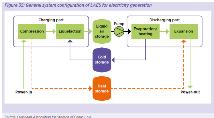
図 II -19 液体空気による蓄熱システム
