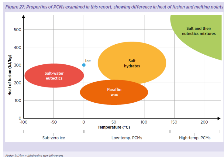
図 II -16 潜熱蓄熱材料の温度領域と材料の関係
