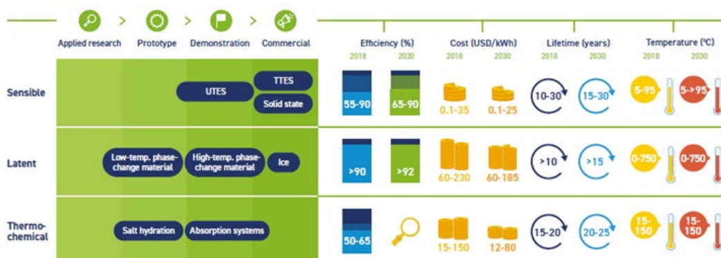
図 II-24 建築物における蓄熱技術開発状況と 2030 年の開発目標 (出典：IRENA, Innovation Outlook Thermal Energy Storage, 2020)
