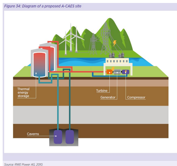
図 II -18 圧縮空気による蓄熱システム
