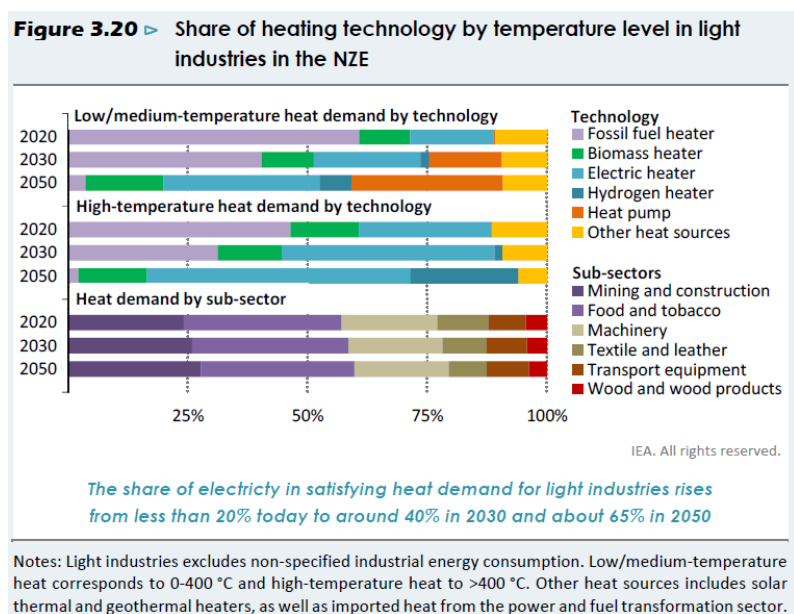
図 II -8 NET ZERO by 2050（NZE）シナリオにおける軽工業部門の温度別の技術シェア （出典：IEA, NET ZERO by 2050, 2021）
